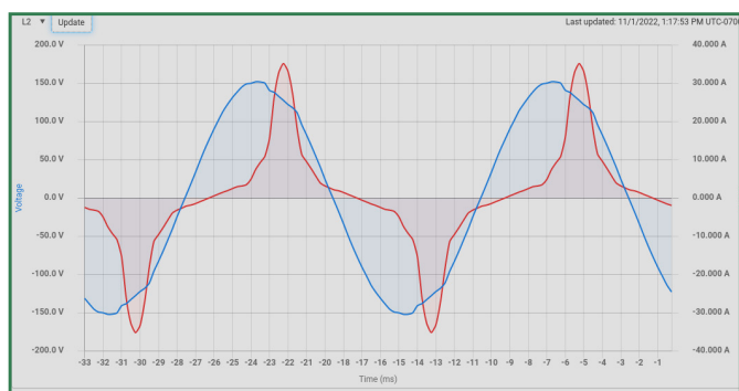
高調波波形の例
