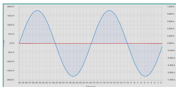
电压骤降示例
